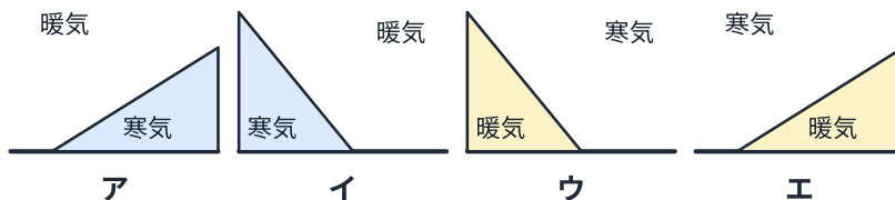
図7 前線付近の空気の様子（断面）
