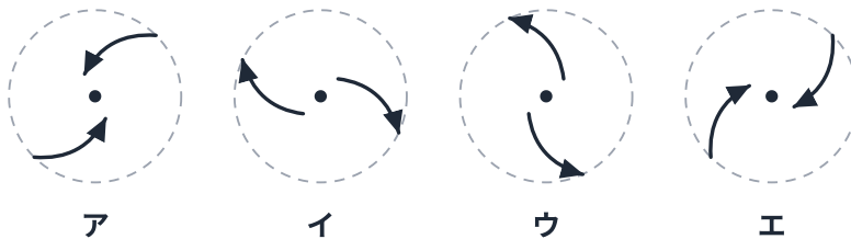
図2 中心付近の風のふき方（上が北）
