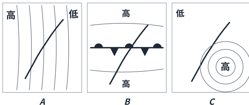
図4 日本付近の天気図（模式図）
