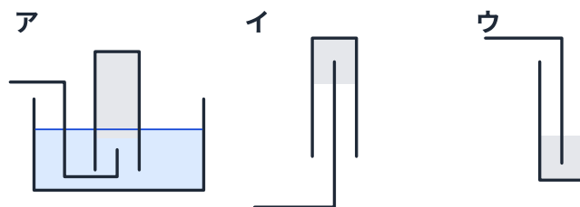
図5 気体を集める3つの方法
