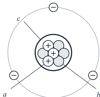
図1 原子のモデル
