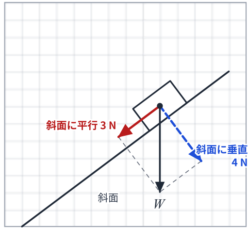
(3) 図4の重力Wの分解 (3点)
